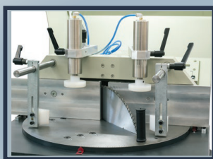
Posição de corte para ângulos menores que 45°.
